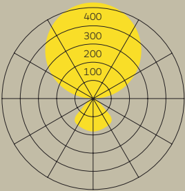
kido 32 140lm/W@4000K
