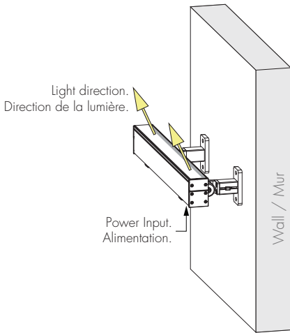
Perspective view, Right feeding side shown, half-frosted lens. Vue de perspective, Côté d'alimentation droite illustré, lentille demi givrée.
